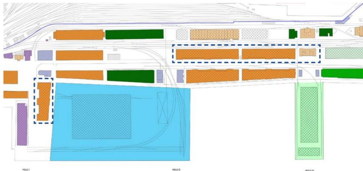
Figura 16 - Bacino II sul quale è ubicato l'Hangar 21 e l'Hangar 22, gemello, ora demolito (EAPT)**
